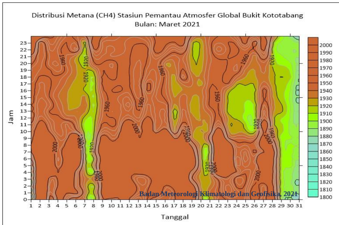
Grafik Diurnal (24 jam) Konsentrasi Metana (CH 4 ) di Bukit Kototabang periode bulan Maret 2021
