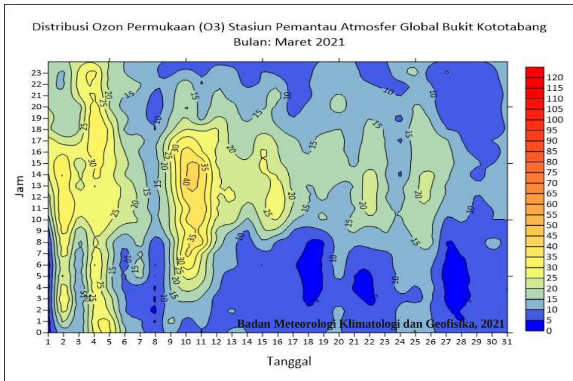
Distribusi Ozon Permukaan ( O_3 ) di Bukit Kototabang periode Maret 2021
