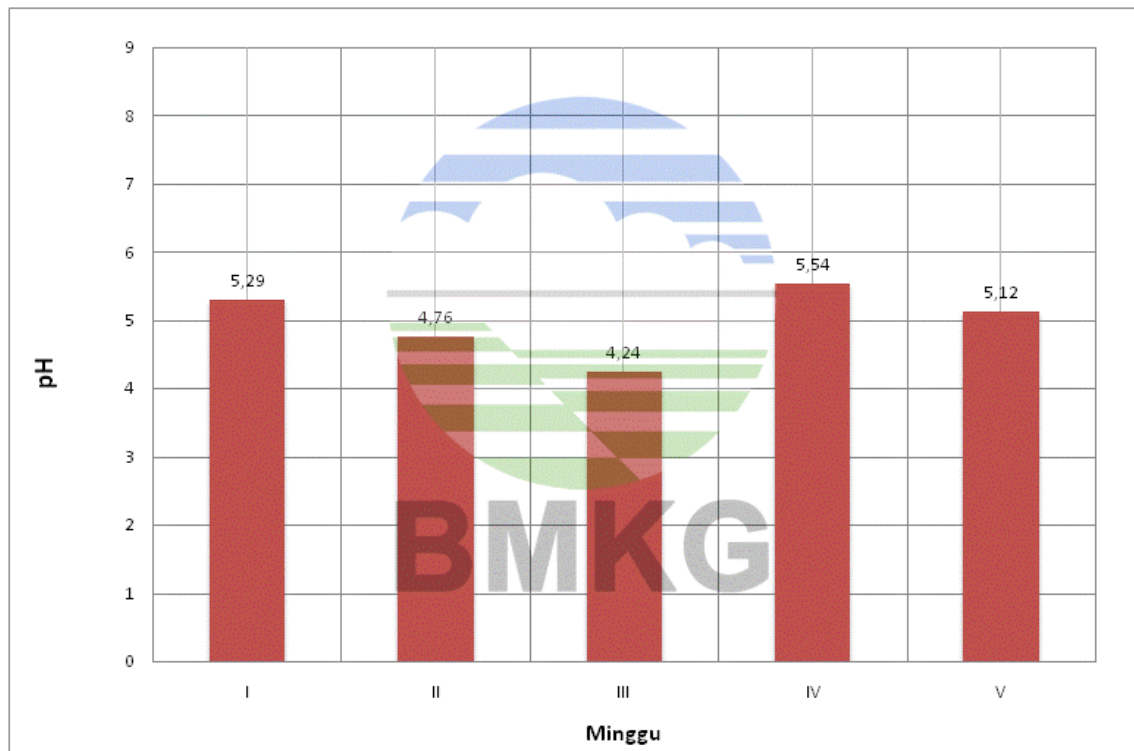
Grafik Tingkat Keasaman (pH) Air Hujan Mingguan dari Penakar Hujan Otomatis (ARG) di Bukit Kototabang periode bulan Maret 2021
