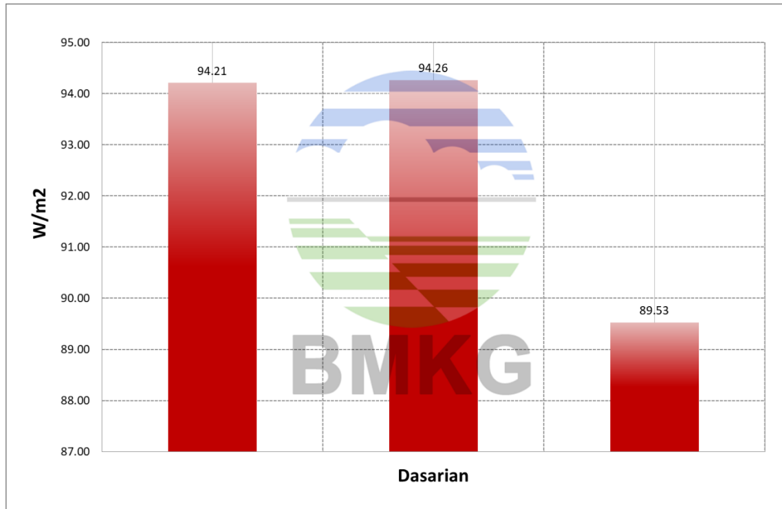
Grafik Dasarian Inframerah di Bukit Kototabang periode bulan Maret 2021
