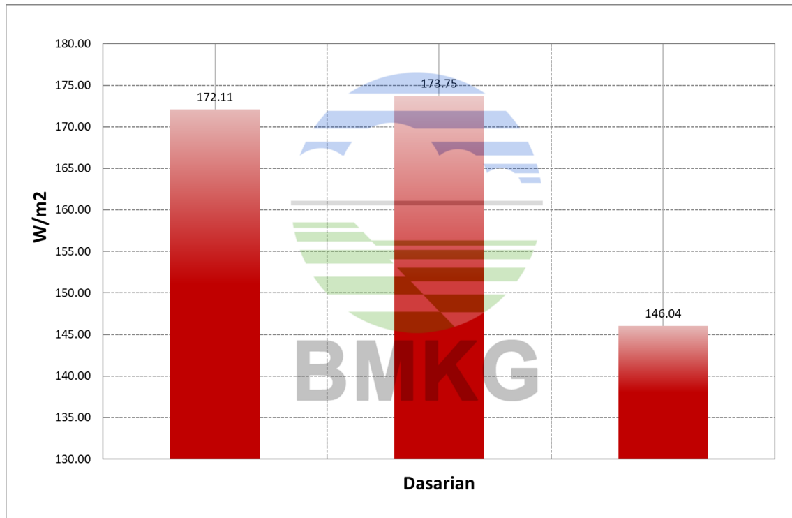
Grafik Dasarian Komponen Global radiasi matahari di Bukit Kototabang periode bulan Maret 2021
