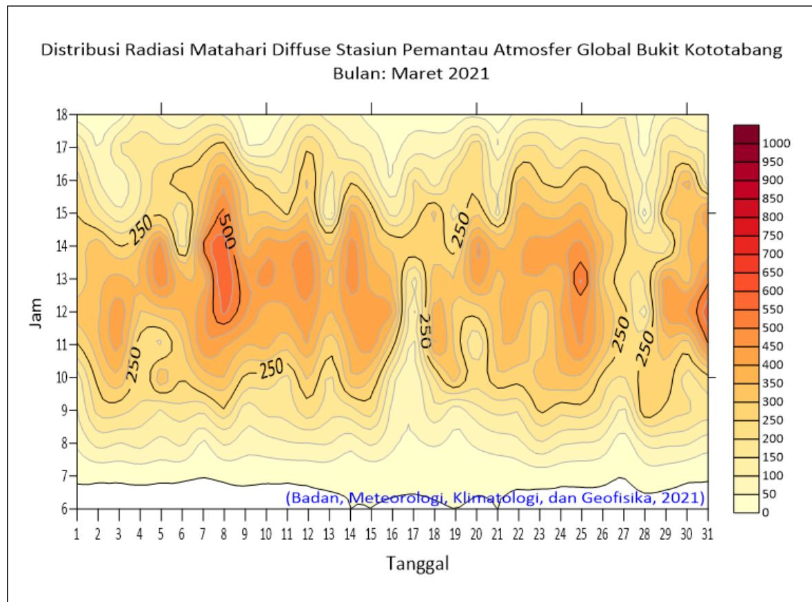
Distribusi Komponen Diffuse Radiasi Matahari di Bukit Kototabang Periode Bulan Maret 2021
