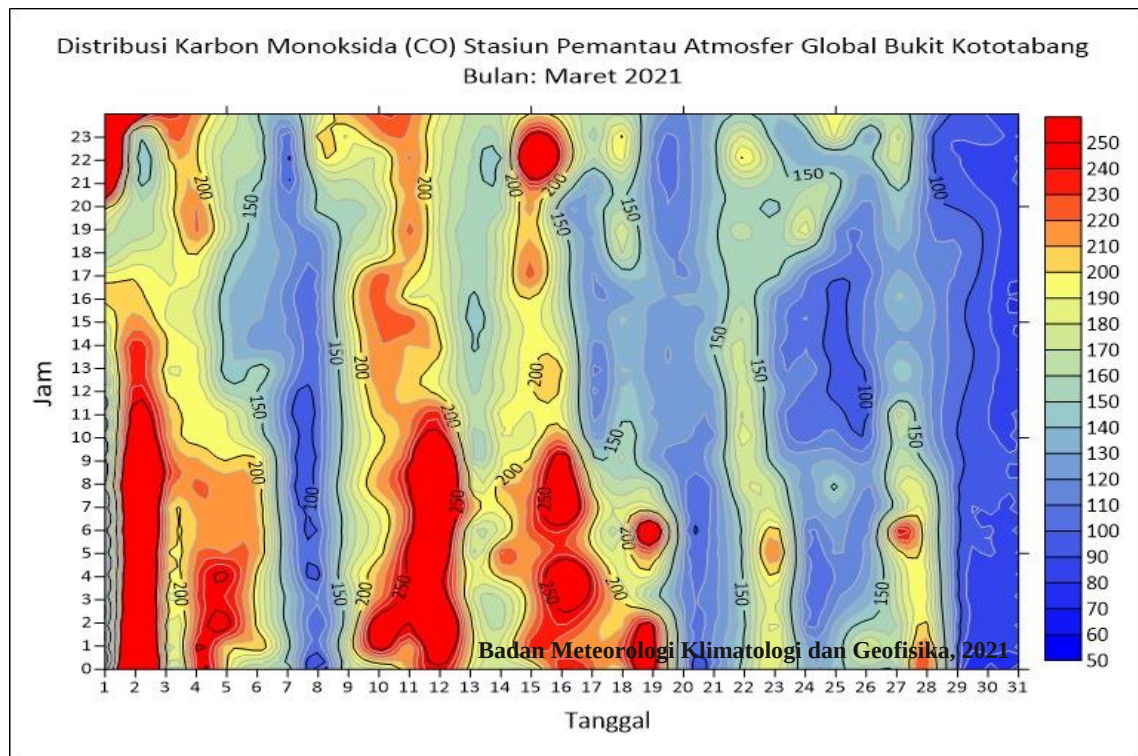
Grafik Diurnal (24 jam) Konsentrasi Karbon Monoksida (CO) di Bukit Kototabang periode bulan Maret 2021
