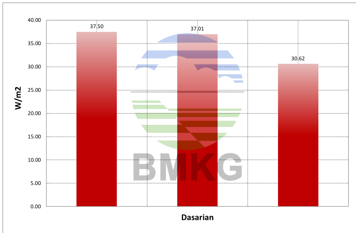
Grafik Dasarian Komponen reflect radiasi matahari di Bukit Kototabang periode bulan Maret 2021
