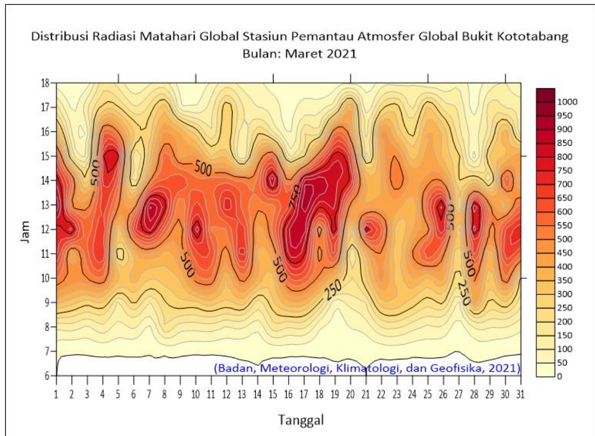
Distribusi Komponen Global Radiasi Matahari di Bukit Kototabang Periode Bulan Maret 2021
