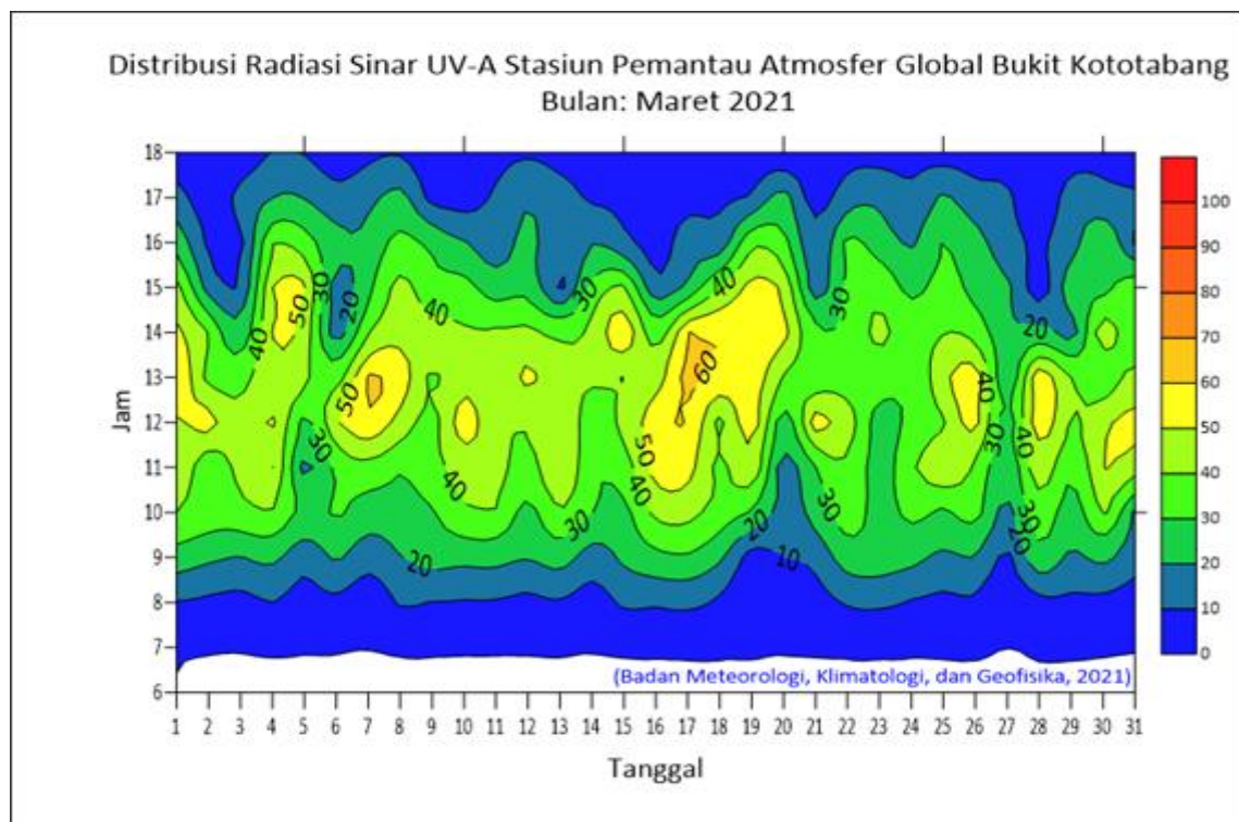
Distribusi Grafik Dasarian Radiasi Sinar UV-A di Bukit Kototabang periode bulan Maret 2021
