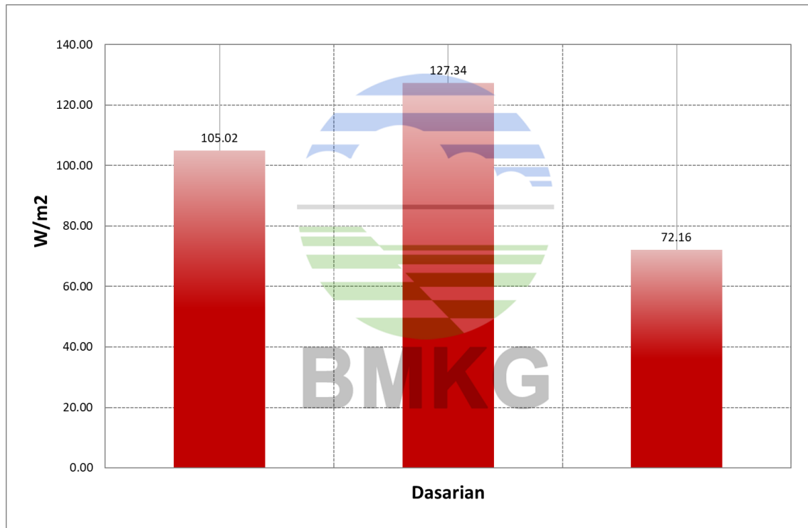
Grafik Dasarian Komponen Direct radiasi matahari di Bukit Kototabang periode bulan Maret 2021
