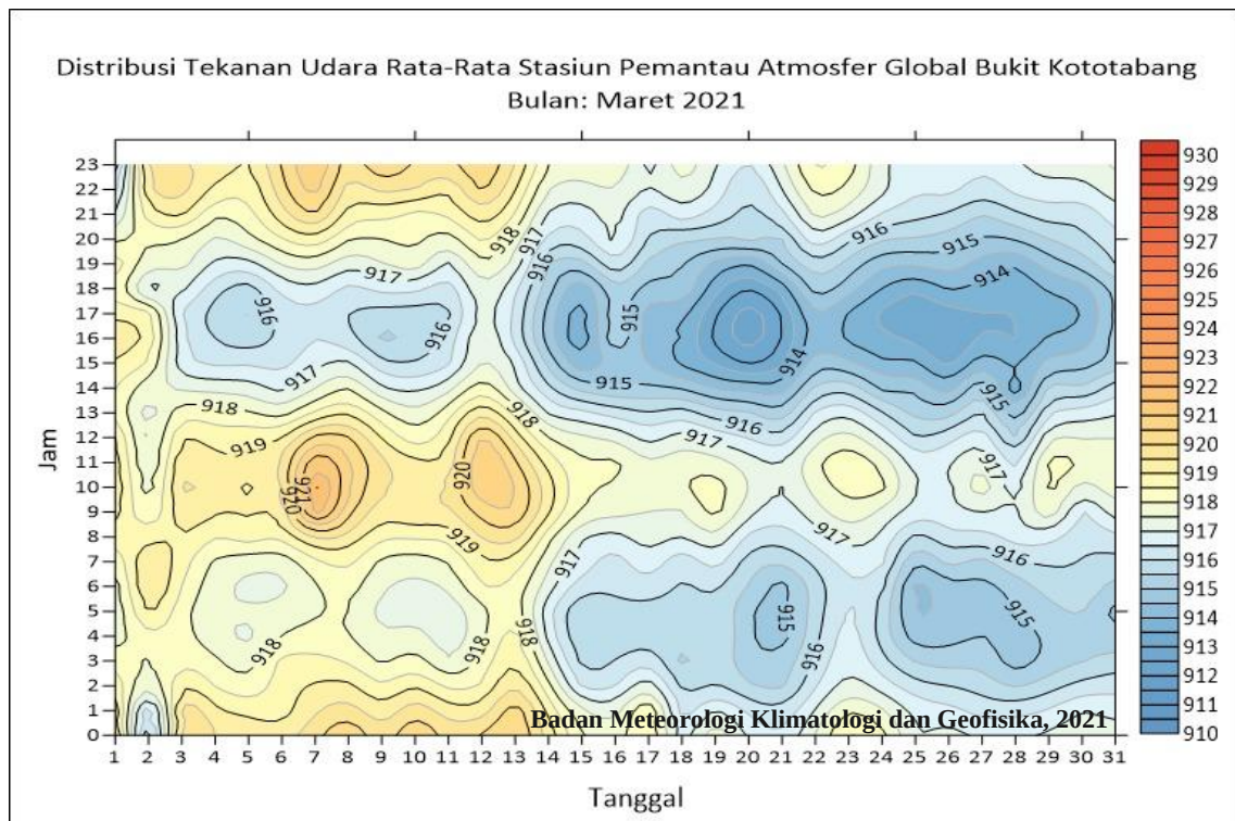
Grafik Harian Tekanan Udara di Bukit Kototabang Bulan Maret 2021
