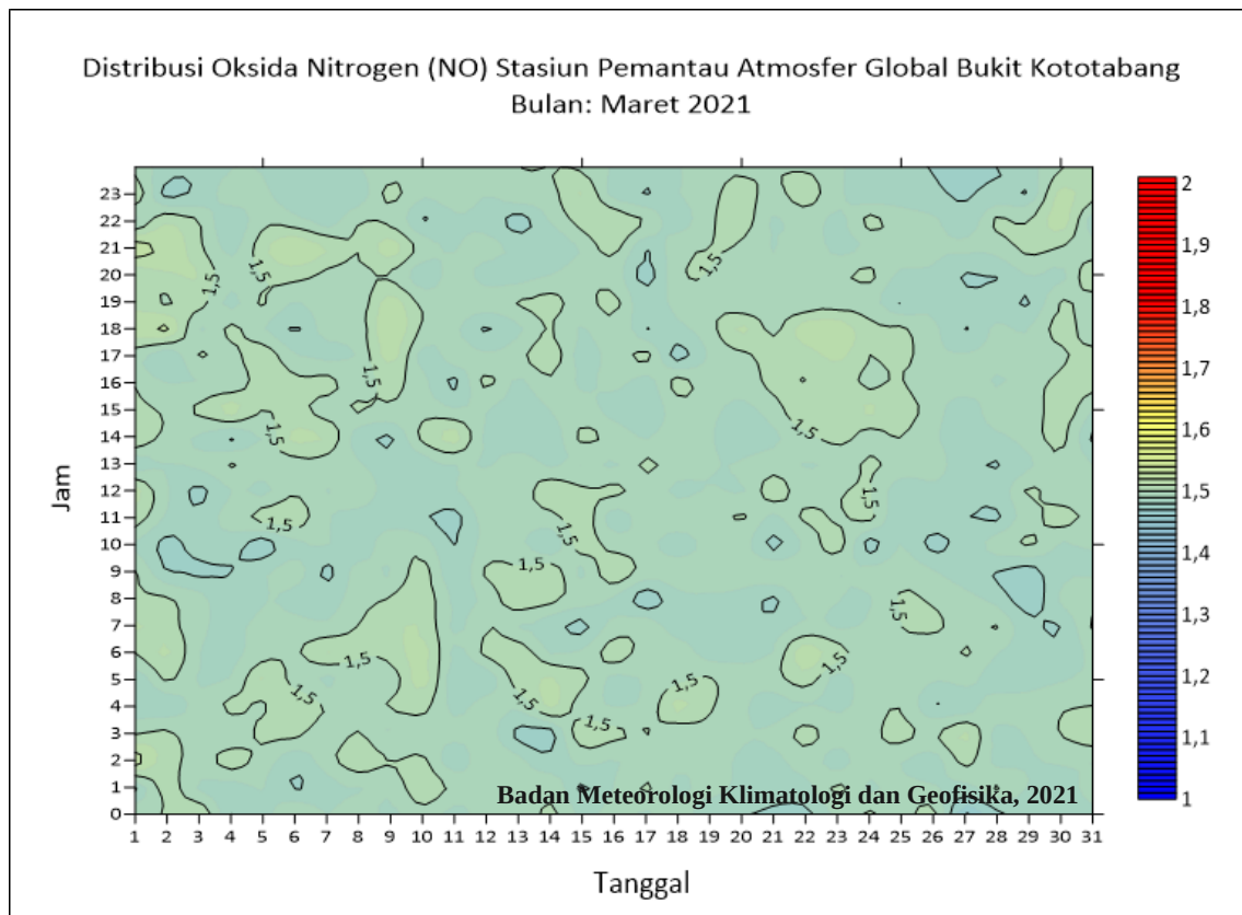
Distribusi Oksida Nitrogen ( \text{NO}_x ) di Bukit Kototabang periode bulan Maret 2021
