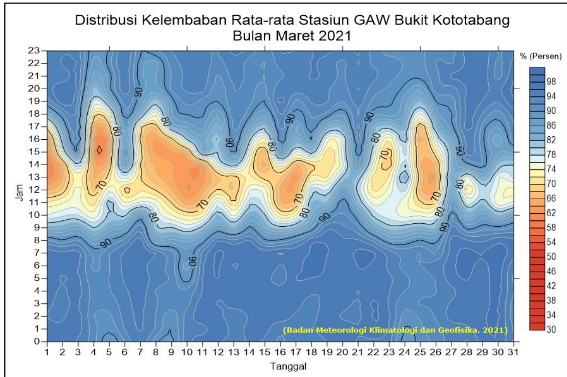
Distribusi sebaran kelembapan udara bulan Maret 2021
