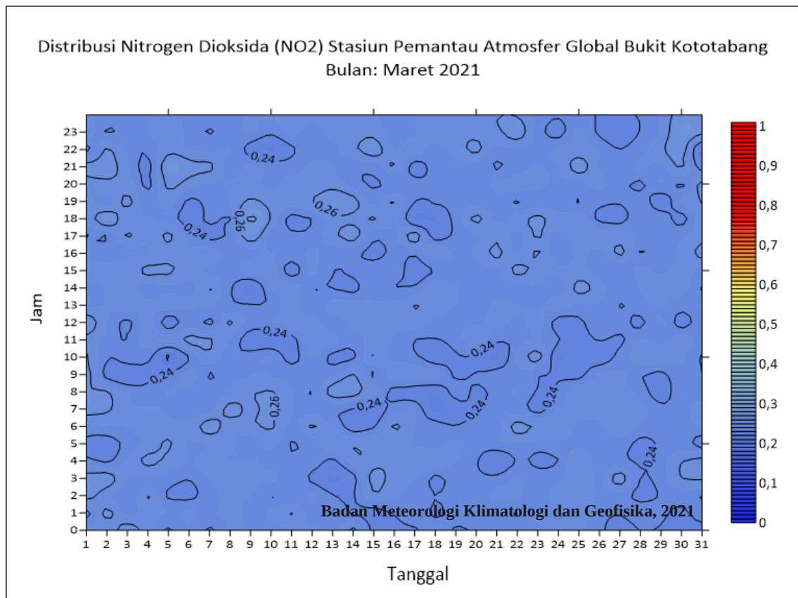
Distribusi Nitrogen Dioksida (NO 2 ) di Bukit Kototabang periode bulan Maret 2021
