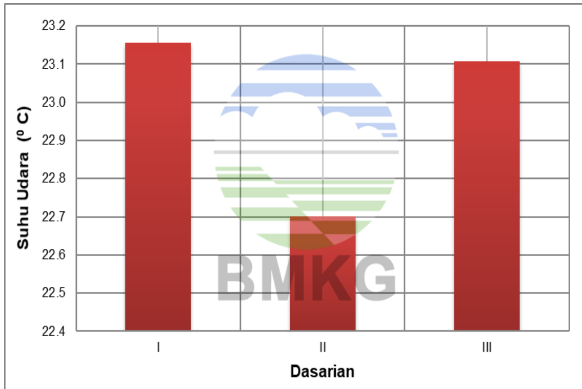
Grafik Dasarian Suhu udara di Bukit Kototabang periode bulan Maret 2021
