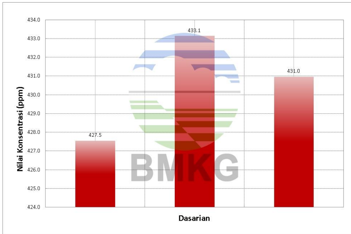
Grafik Dasarian Konsentrasi Karbon Dioksida (CO 2 ) di Bukit Kototabang periode bulan Maret 2021
