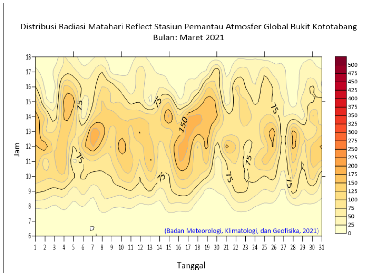
Distribusi Komponen Reflect Radiasi Matahari di Bukit Kototabang Periode Bulan Maret 2021
