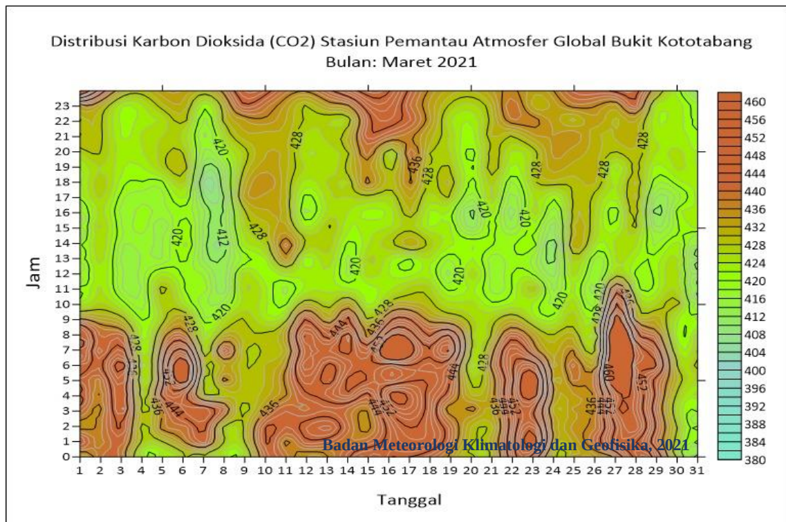
Grafik Diurnal (24 jam) Konsentrasi Karbon Dioksida (CO 2 ) di Bukit Kototabang periode bulan Maret 2021
