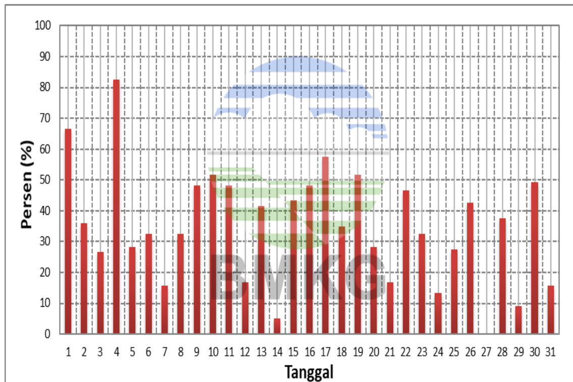
Grafik Harian Lama Penyinaran Matahari di Bukit Kototabang periode bulan Maret 2021
