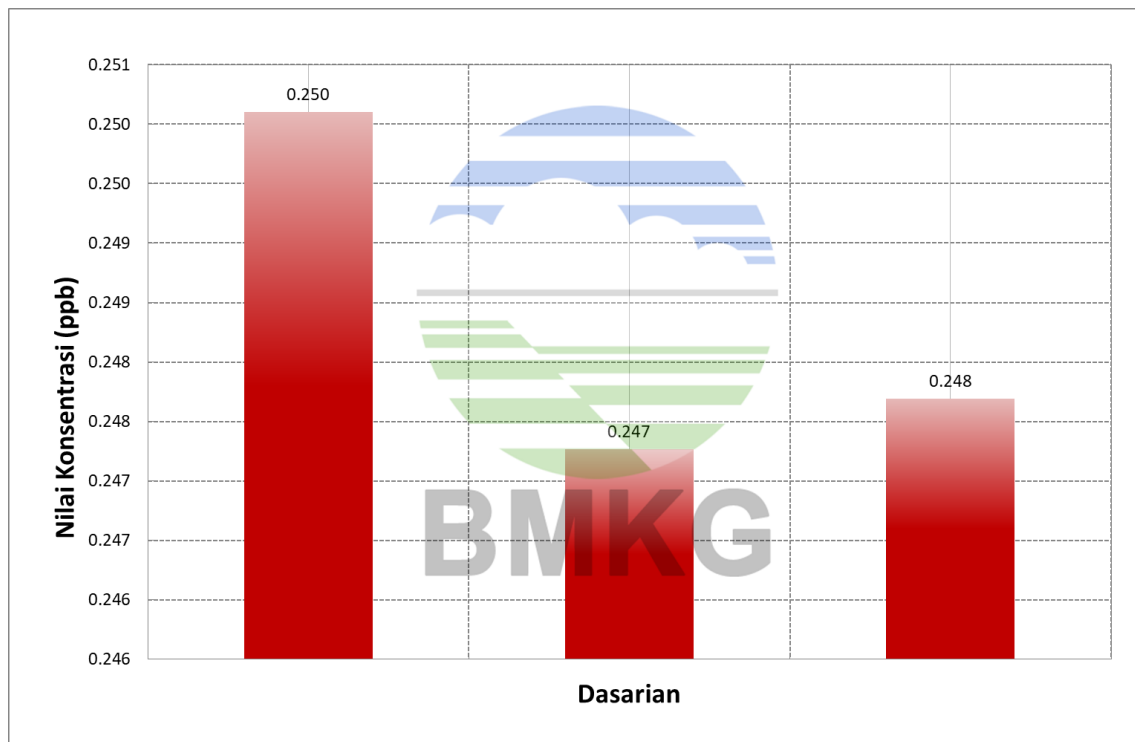
Grafik Dasarian Nitrogen Dioksida ( \text{NO}_2 ) di Bukit Kototabang periode bulan Maret 2021
