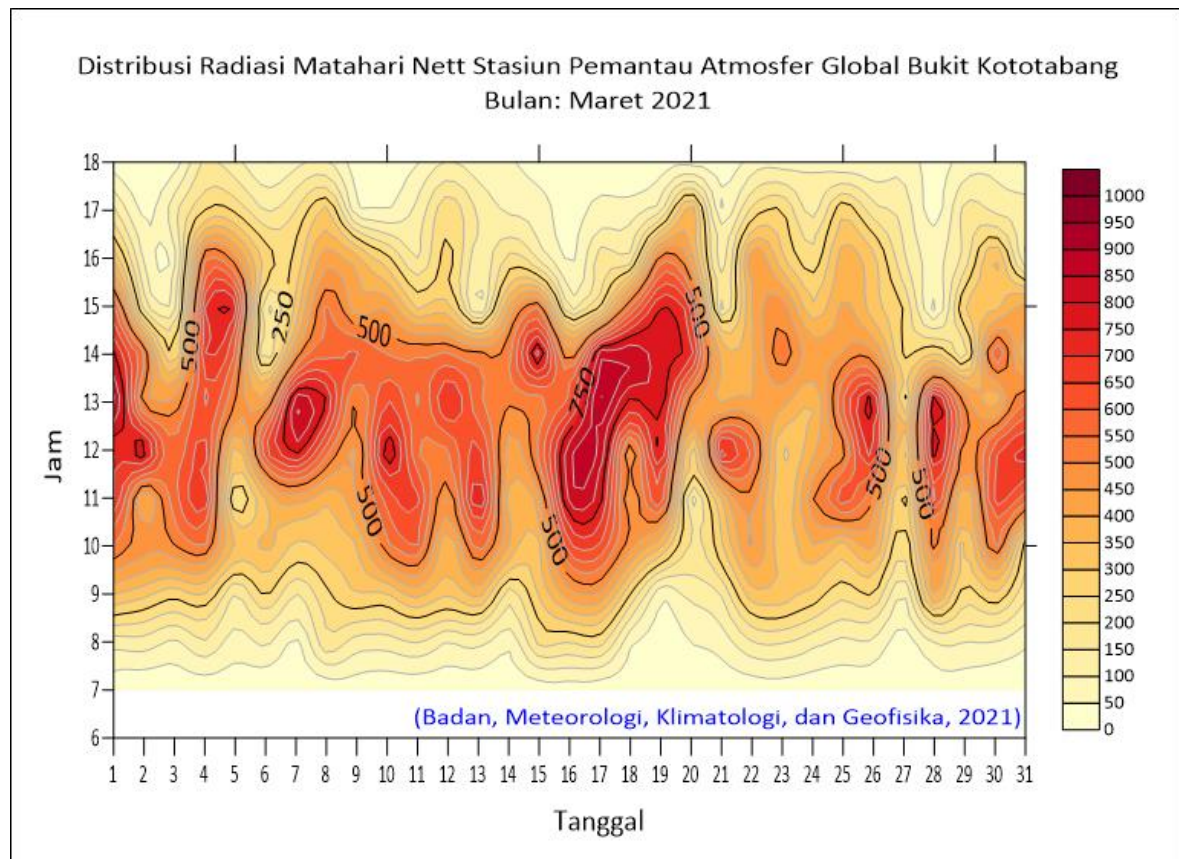
Distribusi Komponen Nett Radiasi Matahari di Bukit Kototabang Periode Bulan Maret 2021
