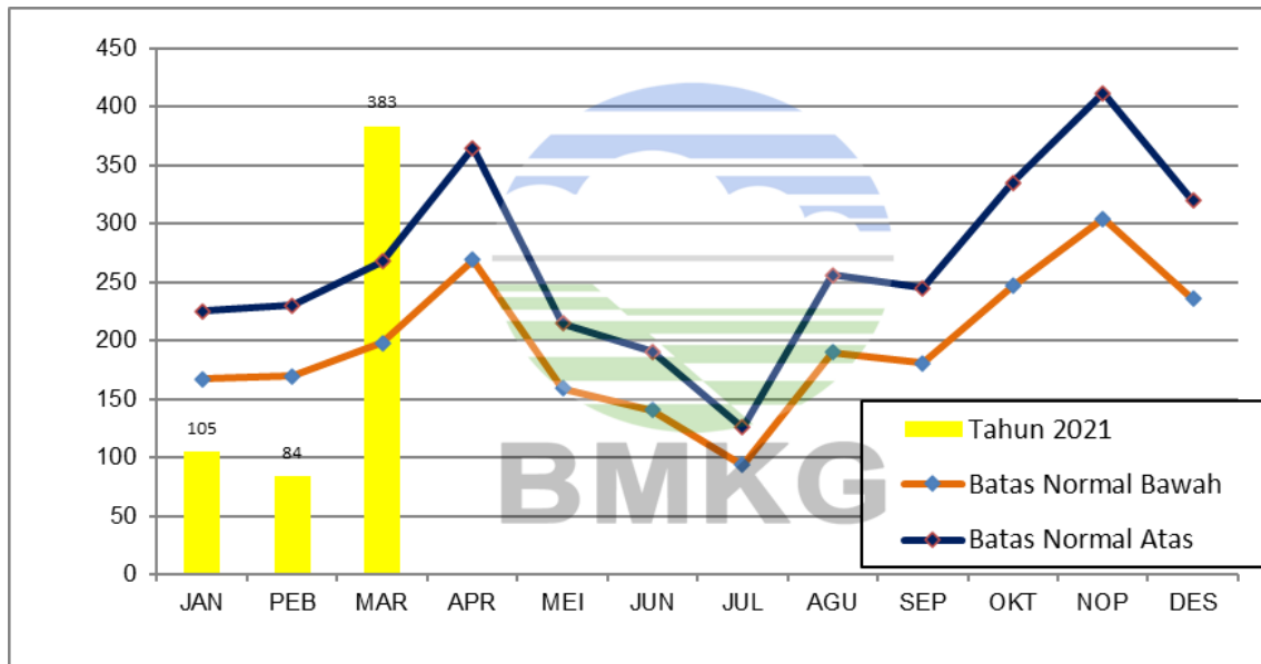
Grafik Curah Hujan Bulanan Bulan Maret 2021
