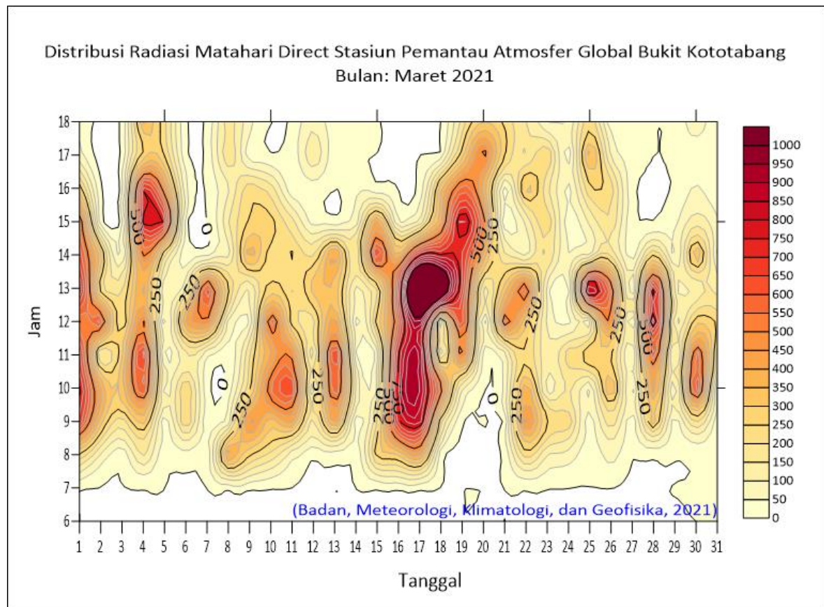
Distribusi Komponen Direct Radiasi Matahari di Bukit Kototabang Periode Bulan Maret 2021
