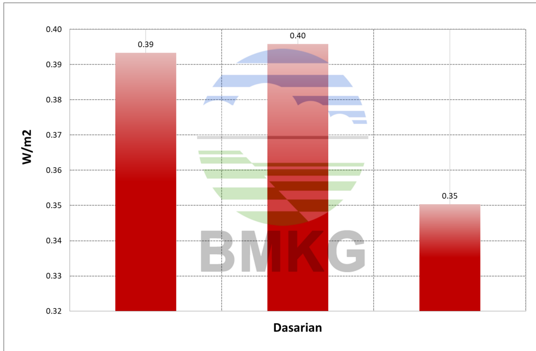
Grafik Dasarian Radiasi Sinar UV-B di Bukit Kototabang periode bulan Maret 2021
