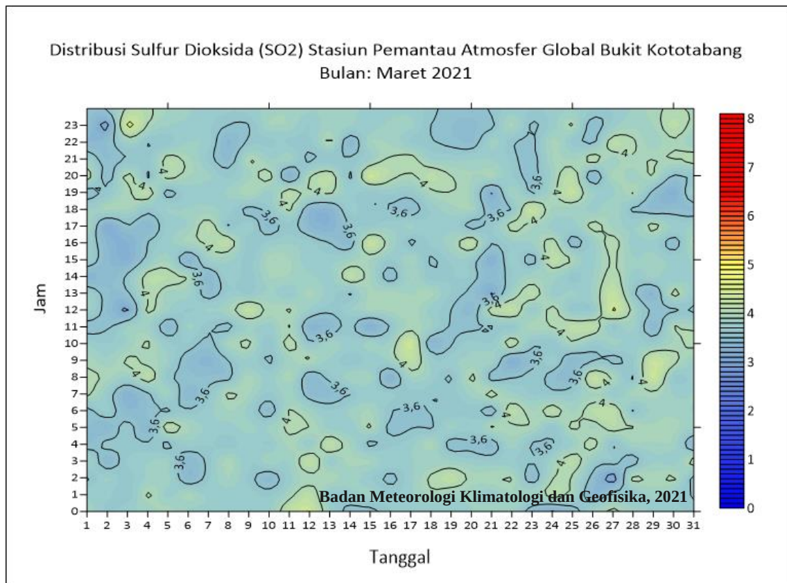
Distribusi Sulfur Dioksida (SO 2 ) di Bukit Kototabang periode bulan Maret 2021
