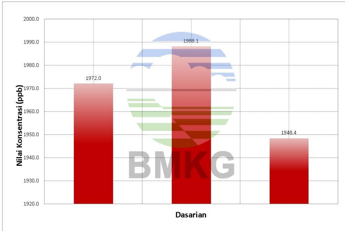
Grafik Dasarian Konsentrasi Metana ( \text{CH}_4 ) di Bukit Kototabang periode bulan Maret 2021
