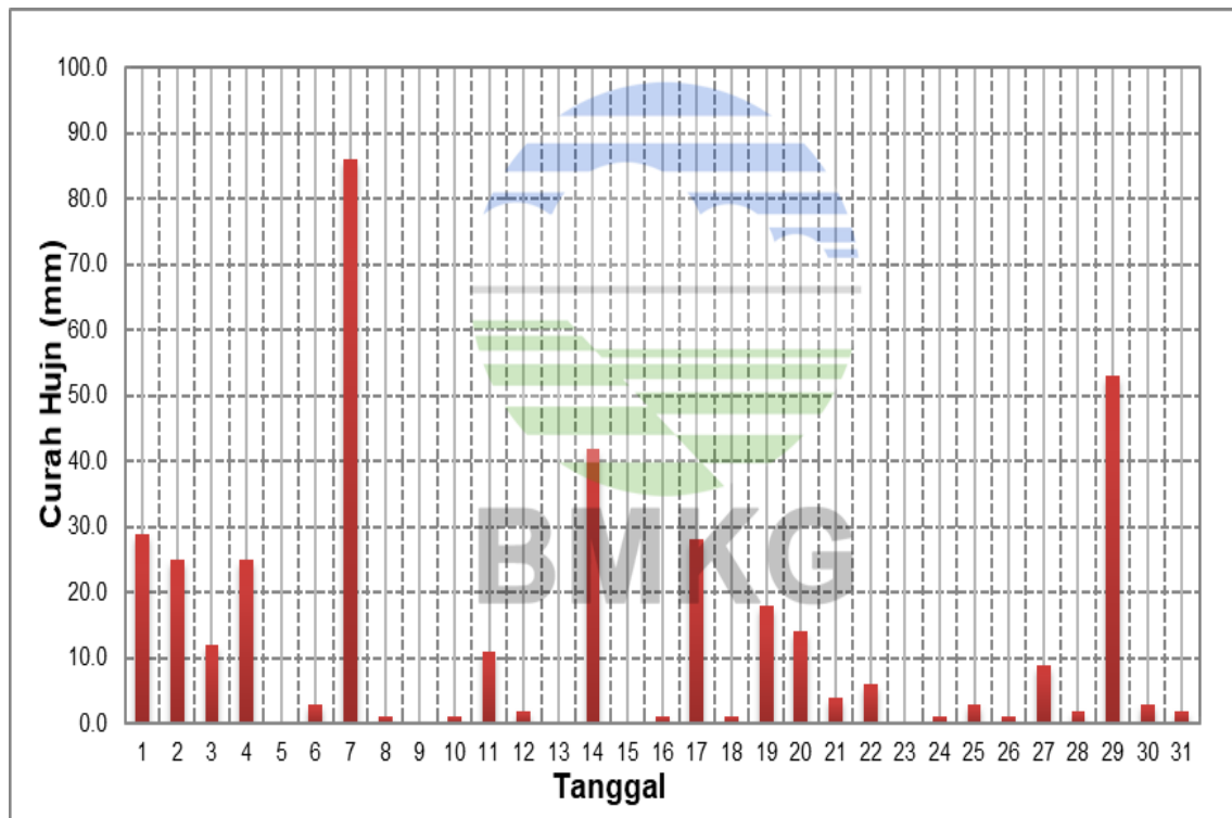
Grafik Curah Hujan Harian Bulan Maret 2021
