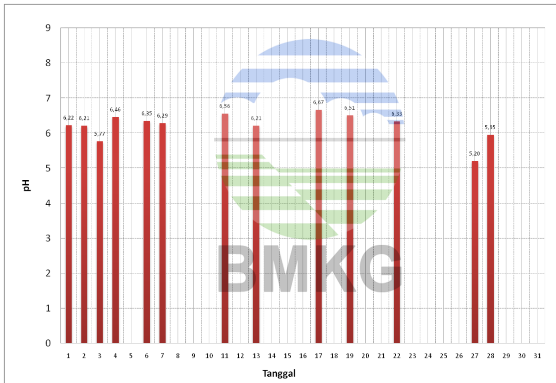
Grafik Tingkat Keasaman (pH) Air Hujan Harian dari Penakar Hujan Observasi (OBS) di Bukit Kototabang periode bulan Maret 2021
