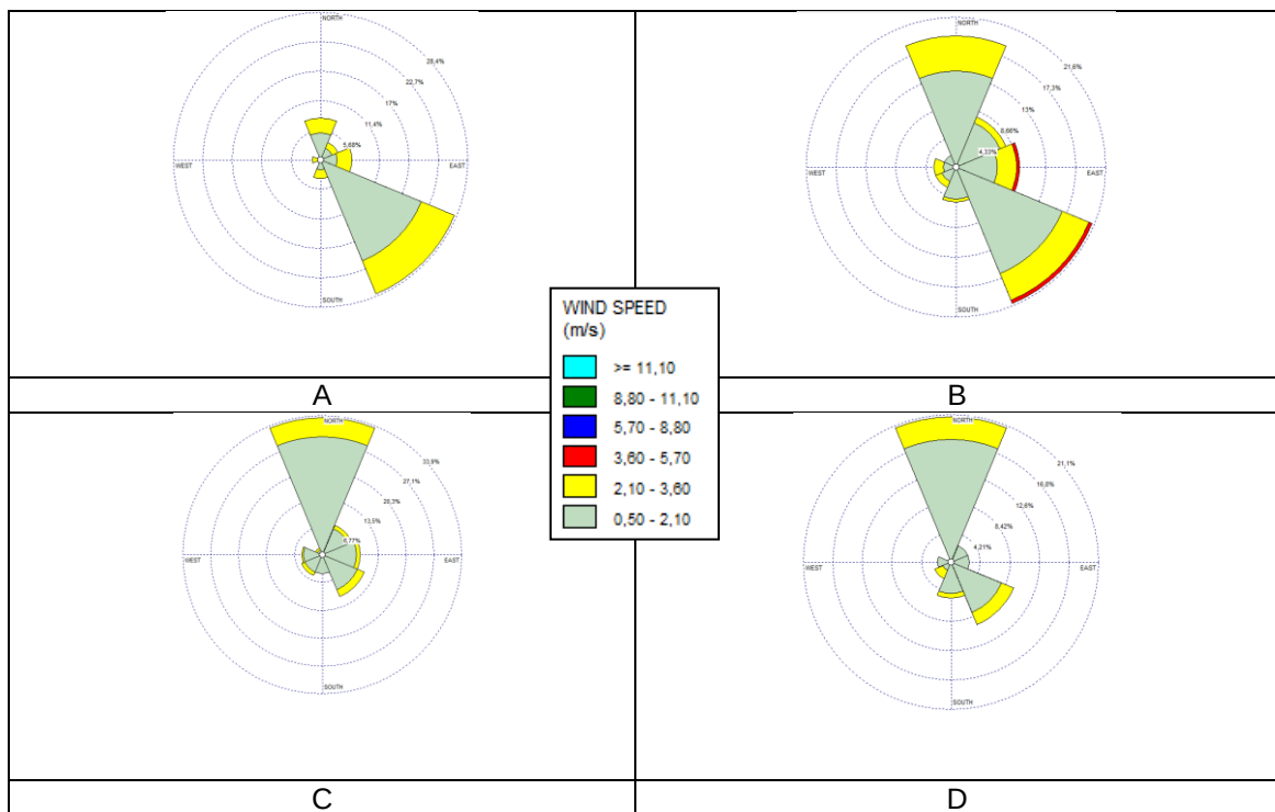
Grafik windrose arah dan kecepatan angin rata-rata pada pukul (a) 00-07 WIB, (b) 07-13 WIB, (c) 13-19 WIB dan (d) 19-23 WIB
