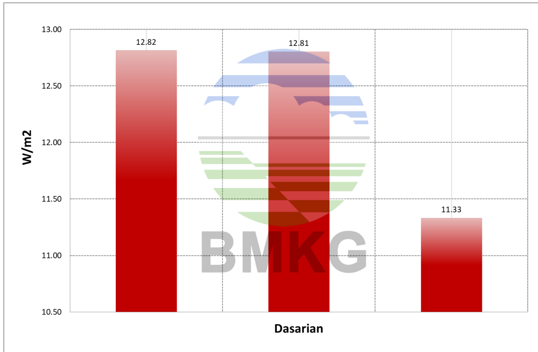
Grafik Dasarian Radiasi Sinar UV-A di Bukit Kototabang periode bulan Maret 2021
