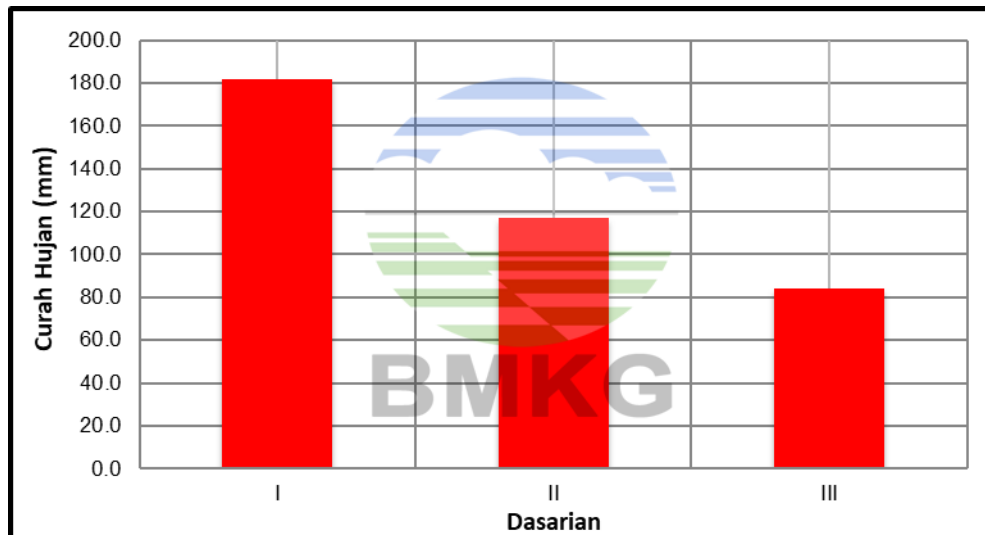
Grafik Curah Hujan Dasarian di Bukit Kototabang bulan Maret 2021
