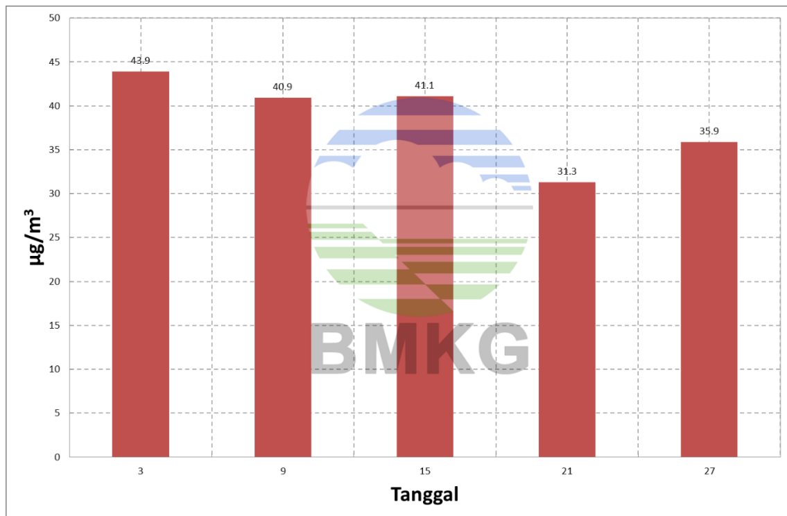
Grafik Konsentrasi SPM di Bukit Kototabang periode bulan Maret 2021
