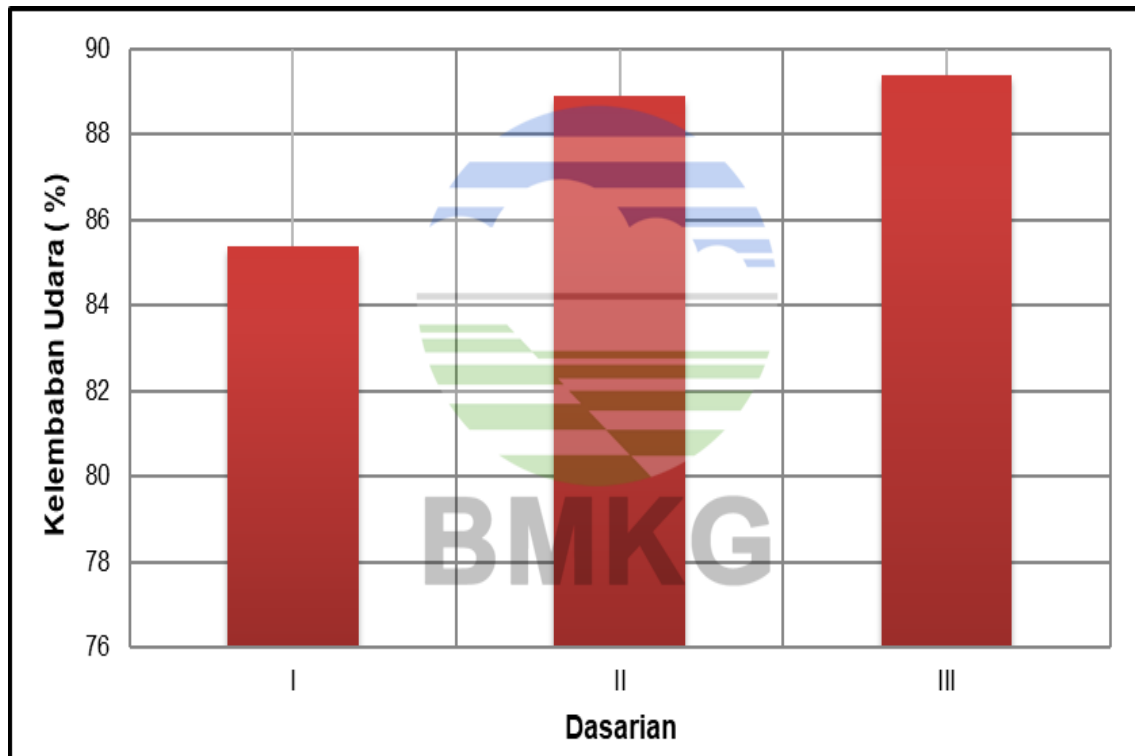
Grafik dasarian kelembapan udara periode bulan Maret 2021
