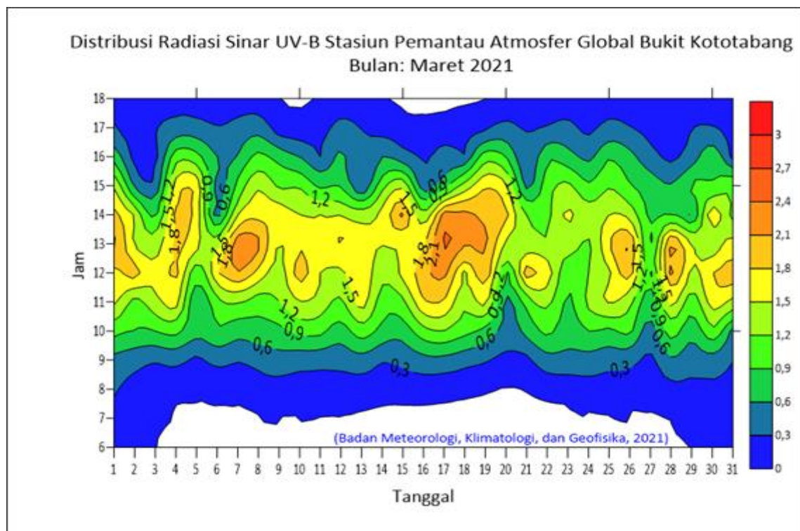
Distribusi Grafik Dasarian Radiasi Sinar UV-B di Bukit Kototabang periode bulan Maret 2021
