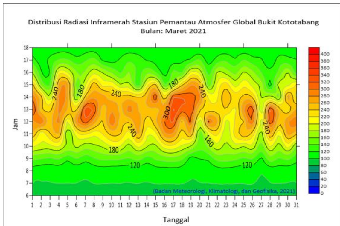
Distribusi Grafik Dasarian Radiasi Inframerah di Bukit Kototabang periode bulan Maret 2021
