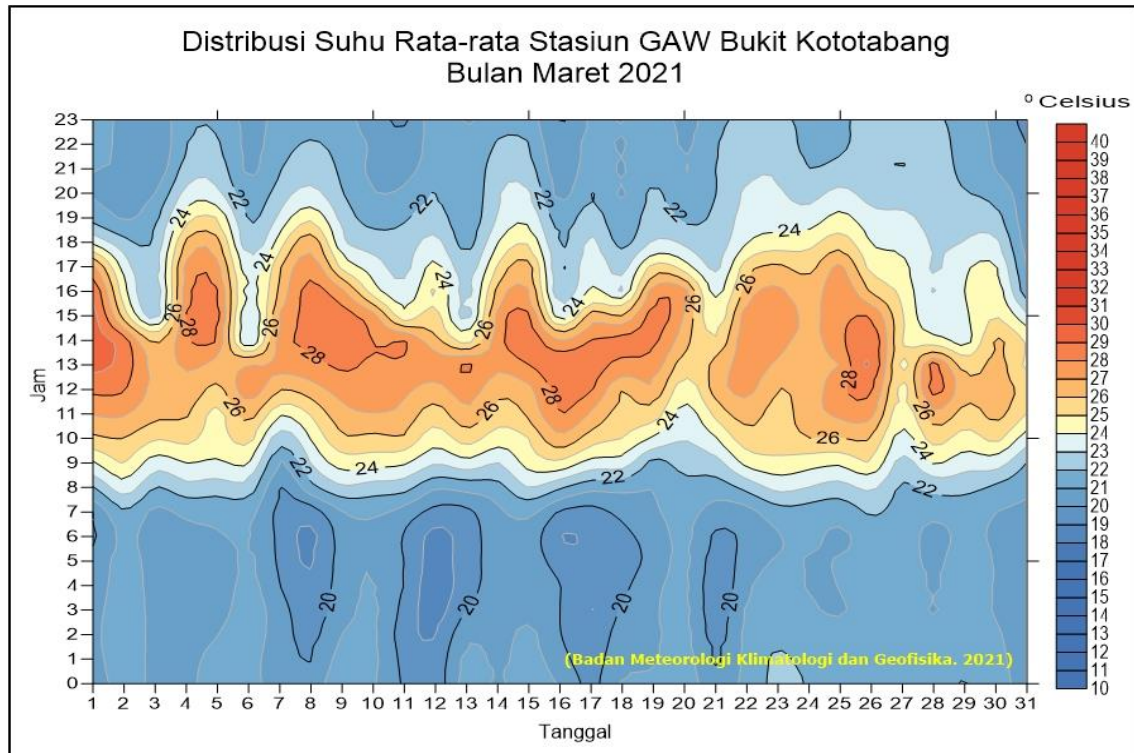
Distribusi suhu udara di Bukit Kototabang periode bulan Maret 2021
