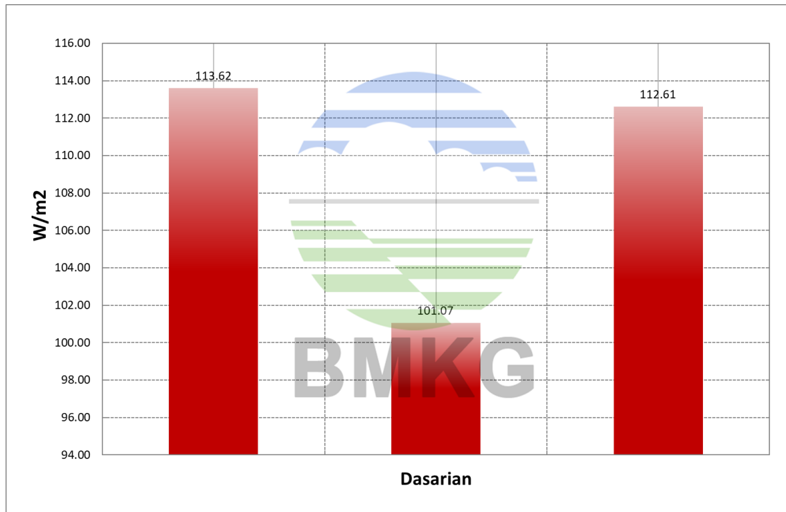
Grafik Dasarian Komponen Diffuse radiasi matahari di Bukit Kototabang periode bulan Maret 2021
