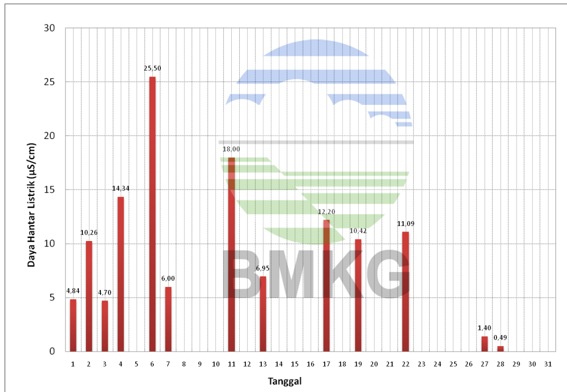
Grafik Daya Hantar Listrik (Conductivity) Air Hujan Harian dari Penakar Hujan Observasi (OBS) di Bukit Kototabang periode bulan Maret 2021
