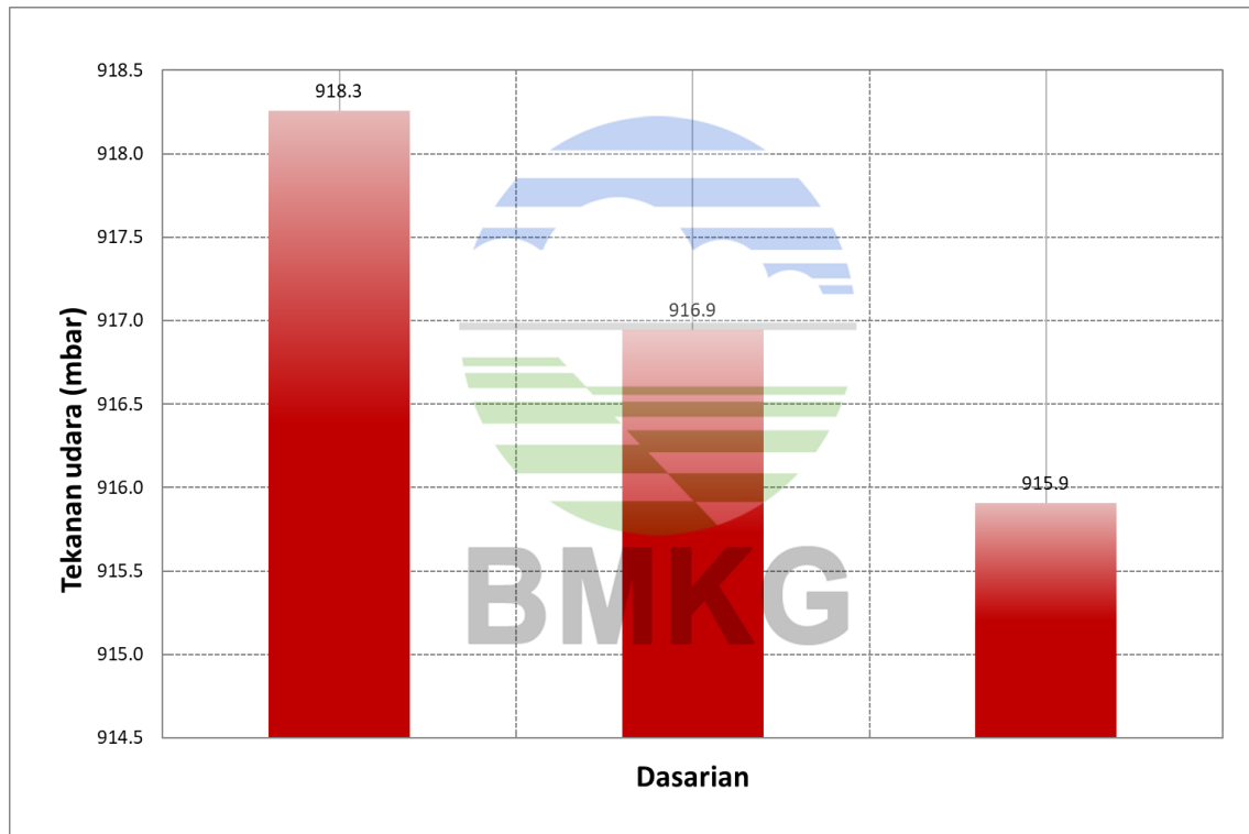
Grafik Dasarian Tekanan Udara di Bukit Kototabang Bulan Maret 2021
