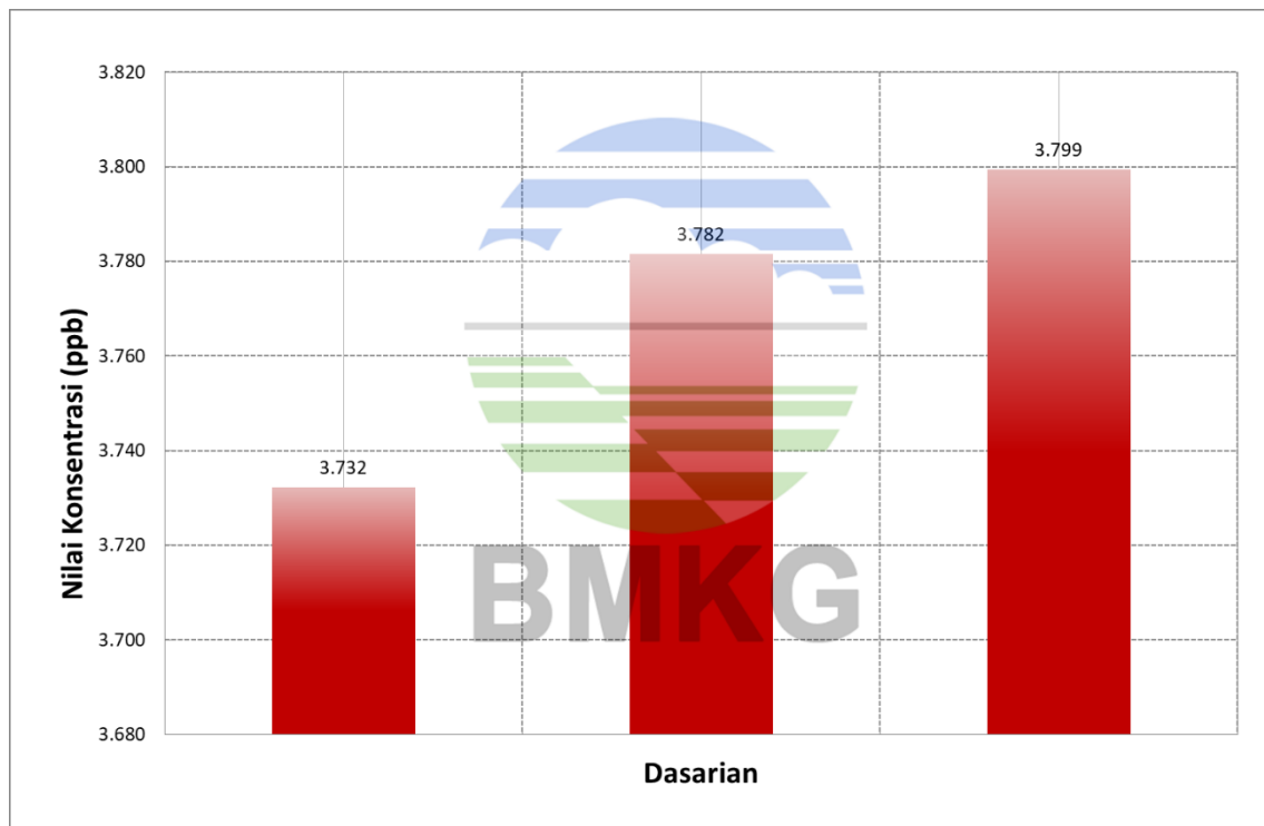
Grafik Dasarian Sulfur Dioksida ( \text{SO}_2 ) di Bukit Kototabang periode bulan Maret 2021
