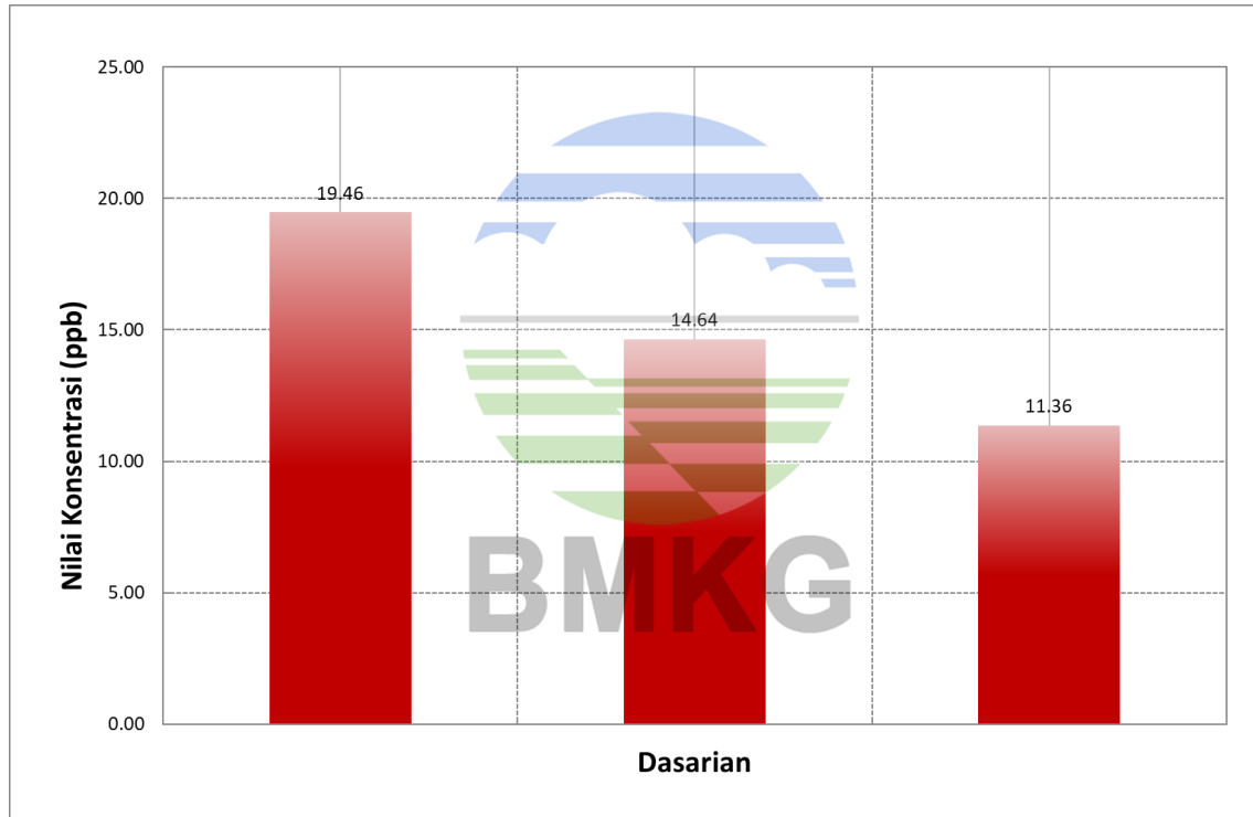
Grafik Dasarian Ozon Permukaan ( O_3 ) di Bukit Kototabang Periode Maret 2021
