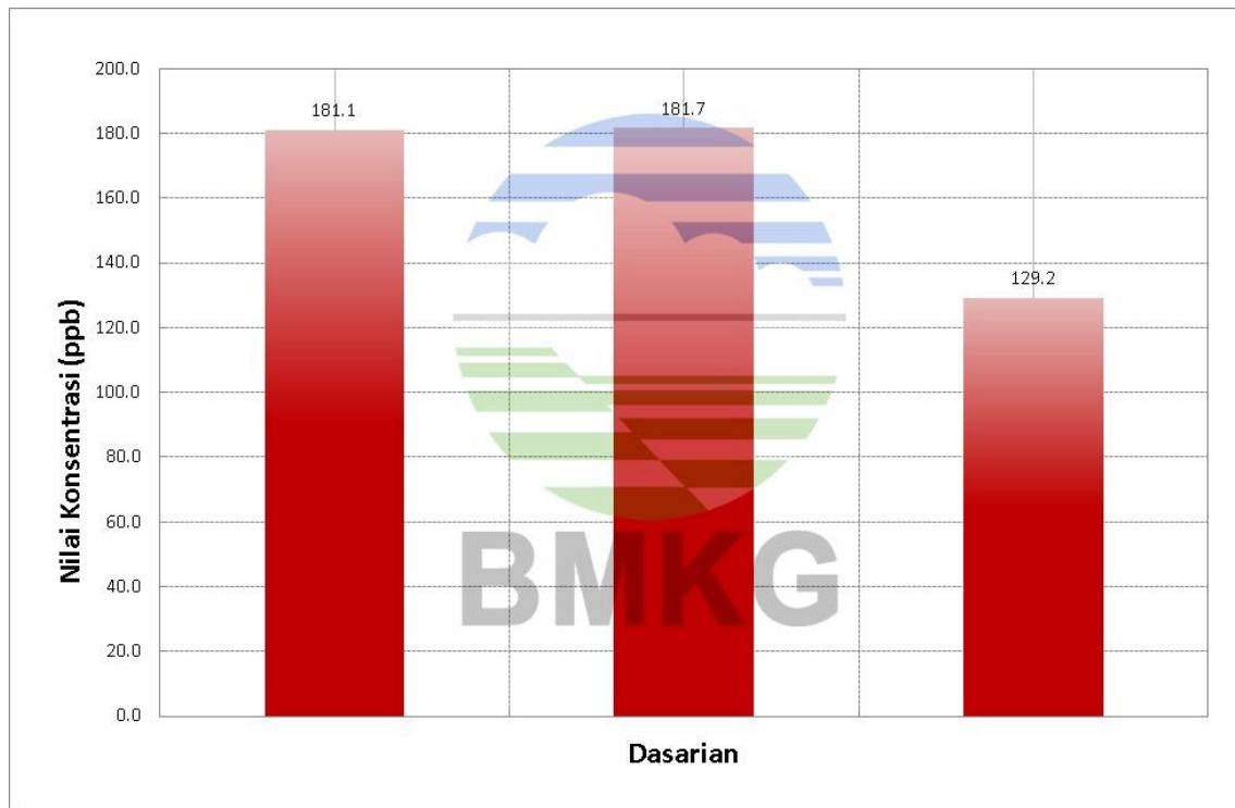
Grafik Dasarian Konsentrasi Karbon Monoksida (CO) di Bukit Kototabang periode bulan Maret 2021
