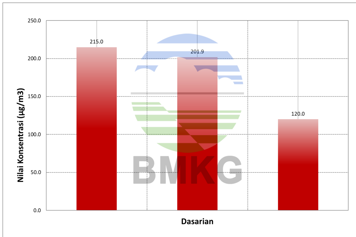
Grafik Dasarian Konsentrasi Black Carbon di Bukit Kototabang periode bulan Maret 2021
