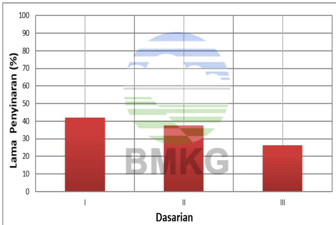
Grafik Dasarian Lama Penyinaran Matahari di Bukit Kototabang periode bulan Maret 2021
