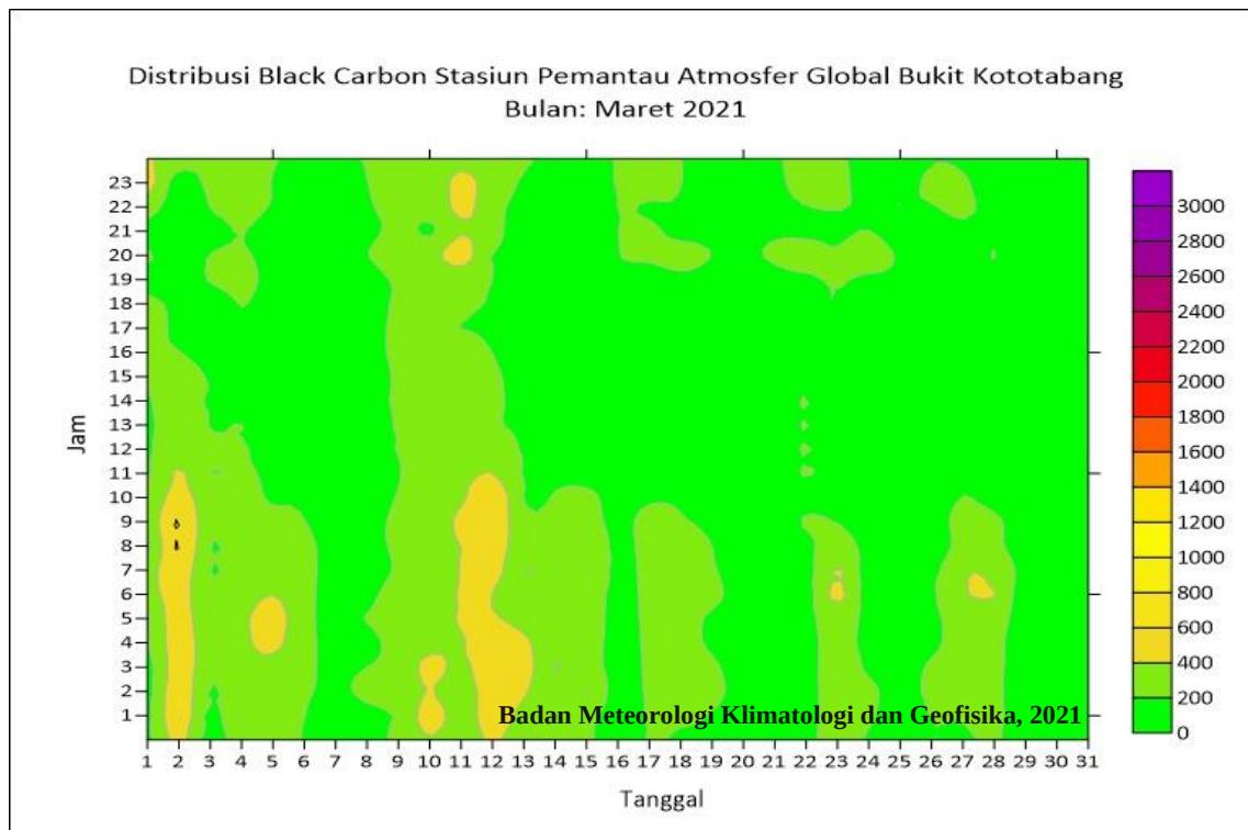
Distribusi Aerosol Black Carbon di Bukit Kototabang periode bulan Maret 2021
