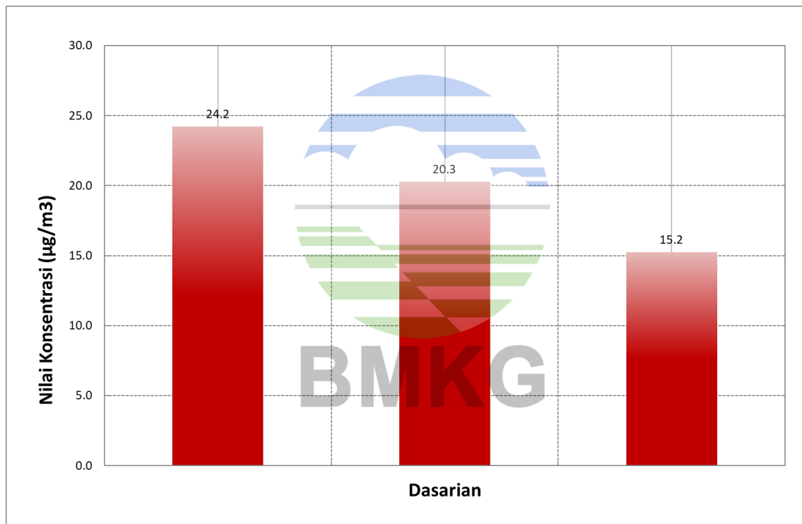
Grafik Rata-rata Dasarian Konsentrasi PM-10 di Bukit Kototabang periode bulan Maret 2021
