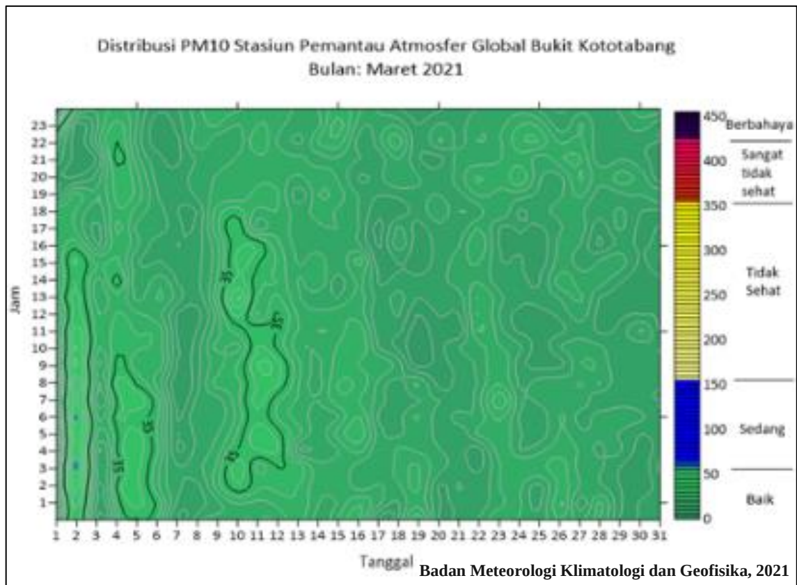
Distribusi konsentrasi PM10 pada bulan Maret 2021
