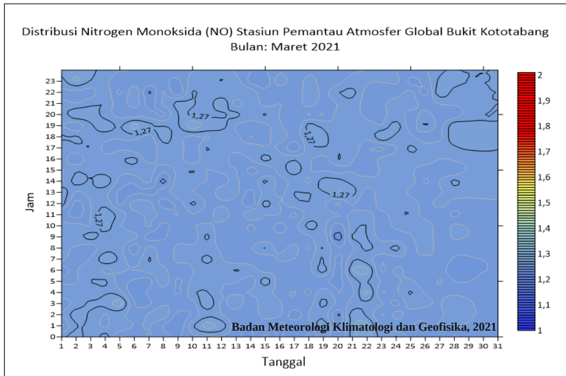
Distribusi Nitrogen monoksida (NO) di Bukit Kototabang periode bulan Maret 2021
