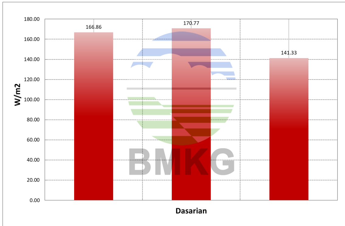
Grafik Dasarian Komponen Nett radiasi matahari di Bukit Kototabang periode bulan Maret 2021
